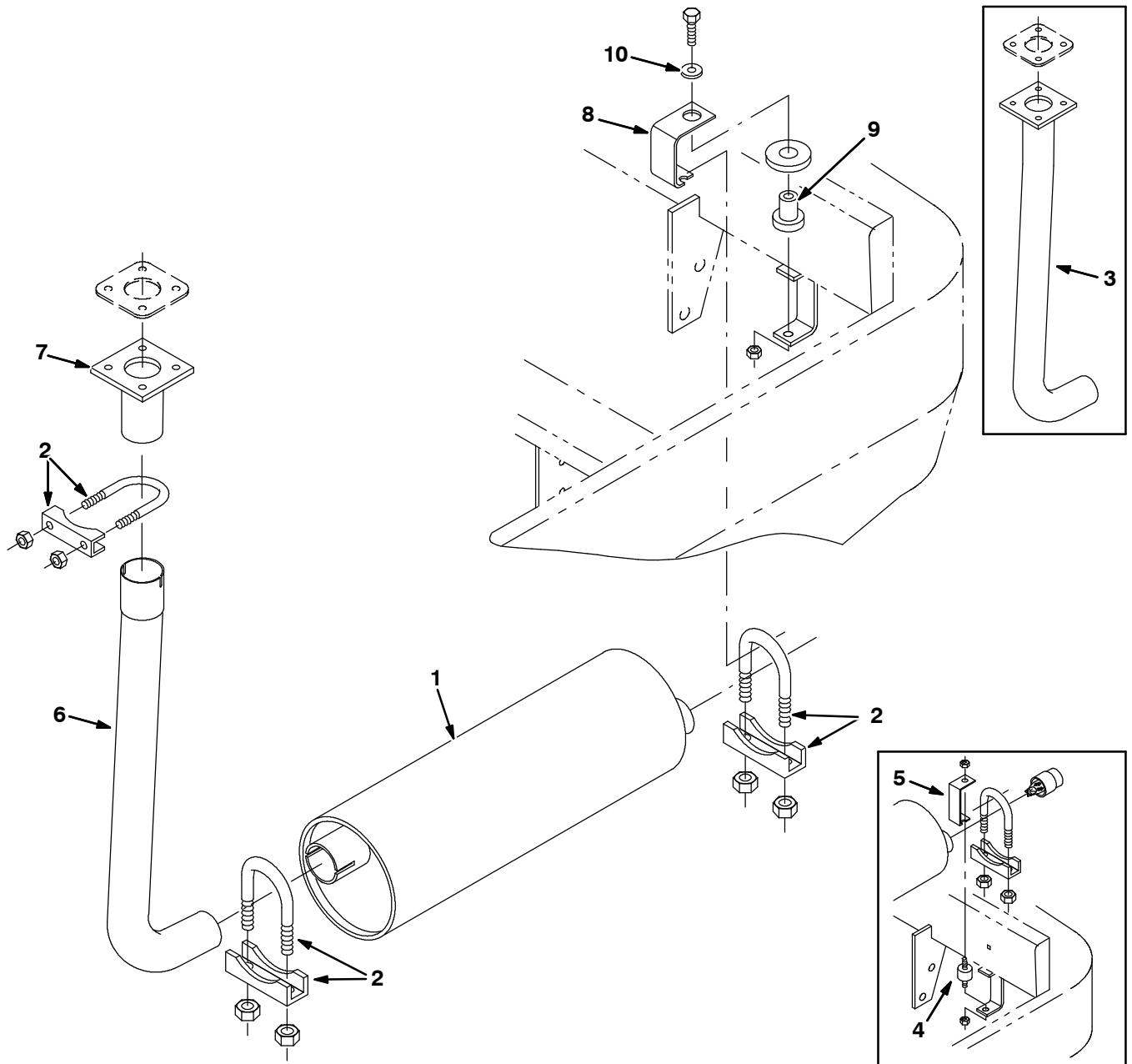
Fig. 20 - Muffler Group
