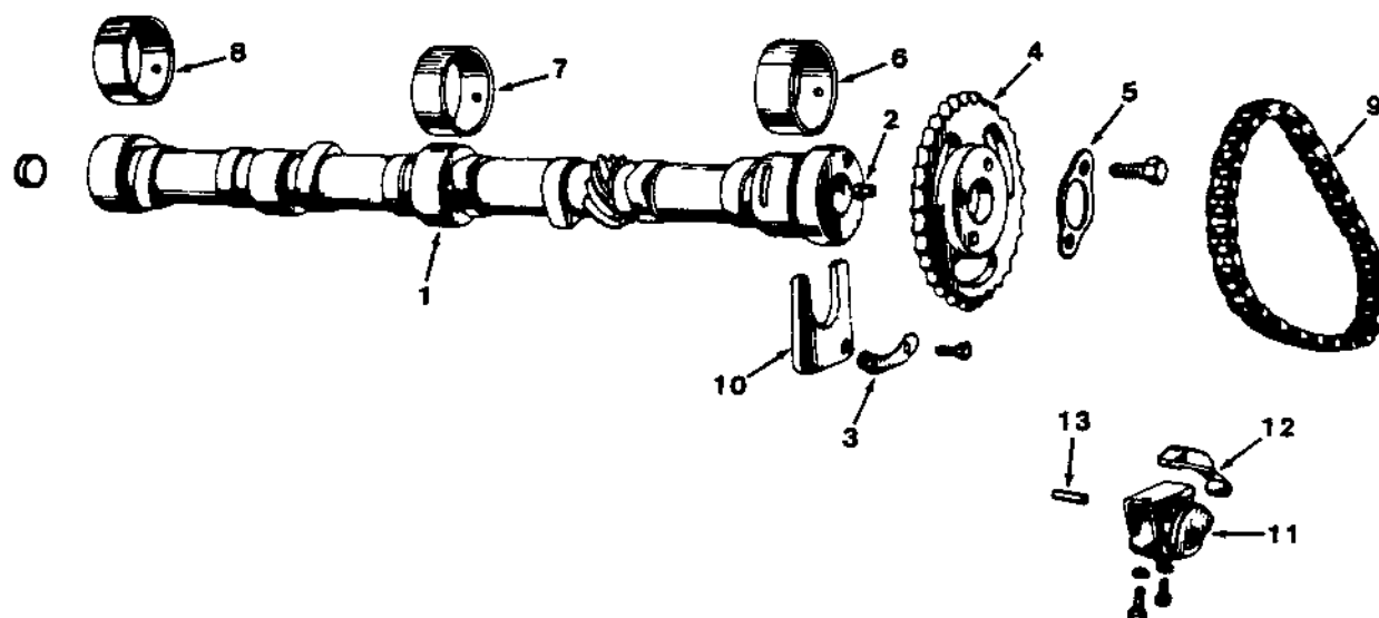
Fig. 4 - Camshaft Group
