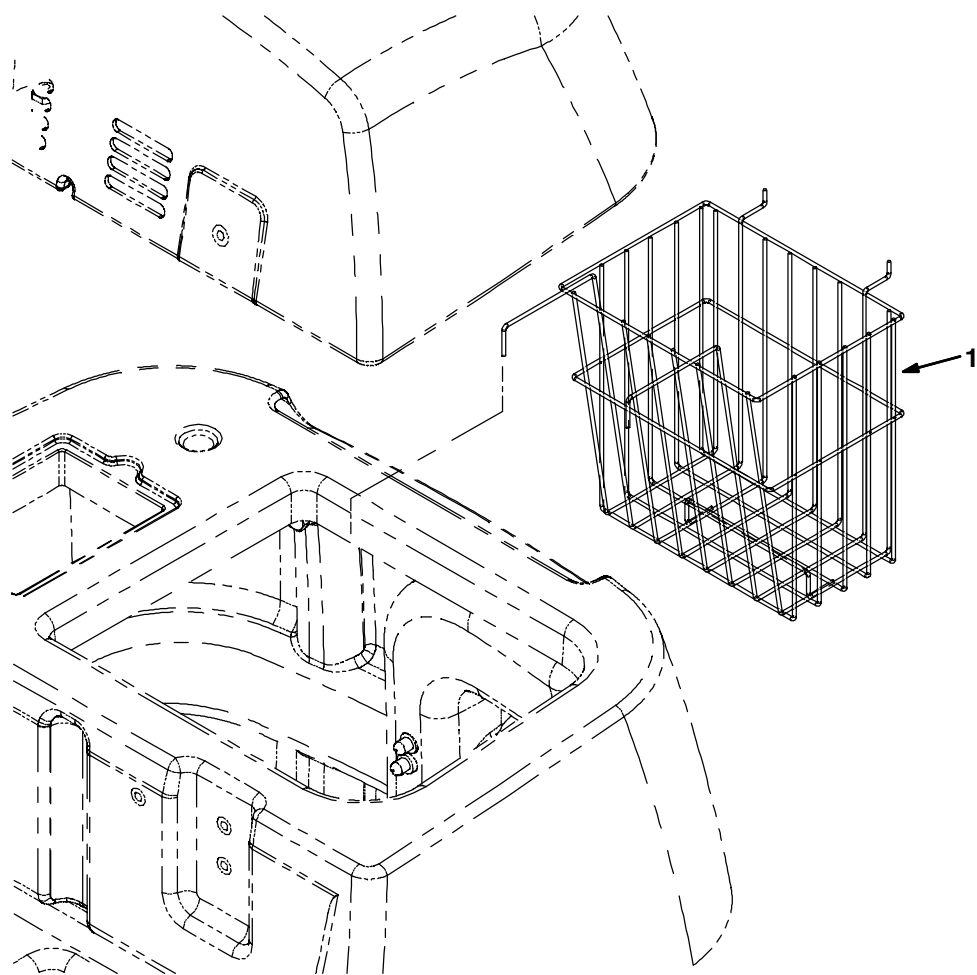
Fig. 4 - Basket Kit
